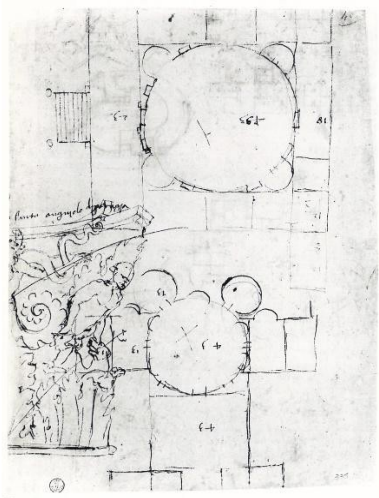
Francesco Di Giorgio Martini, Schizzo delle Piccole Terme , s.d.
